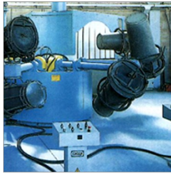
Formowanie rotacyjne
