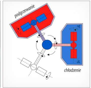
Formowanie rotacyjne
