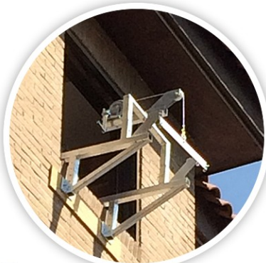
Konstrukcja nośna
